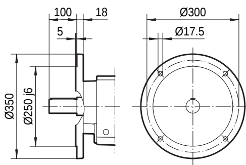
II Ø350
