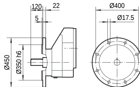
II Ø450
